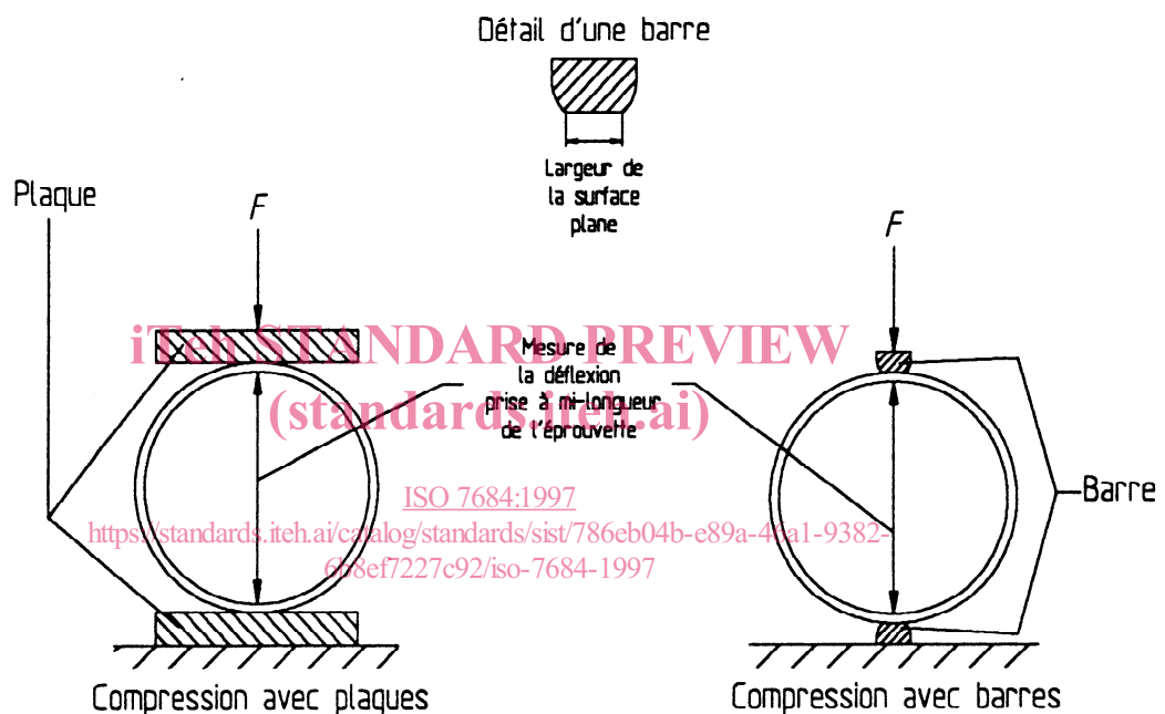
Figure 1 - Schéma de l'appareillage
