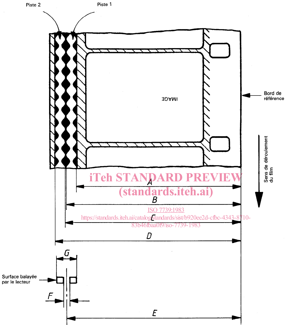
Figure — Double piste sonore optique sur copie d'exploitation cinématographique 16 mm
