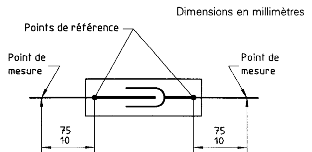
Figure 6 — Résistance de contact — Raccordement câble à câble
