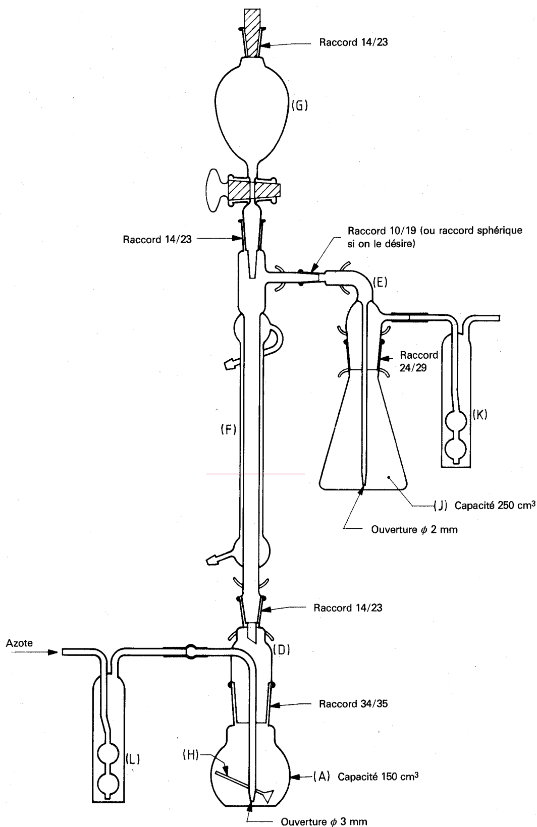
Figure 2 — Appareil type pour la production et l'absorption de l'hydrogène sulfuré
