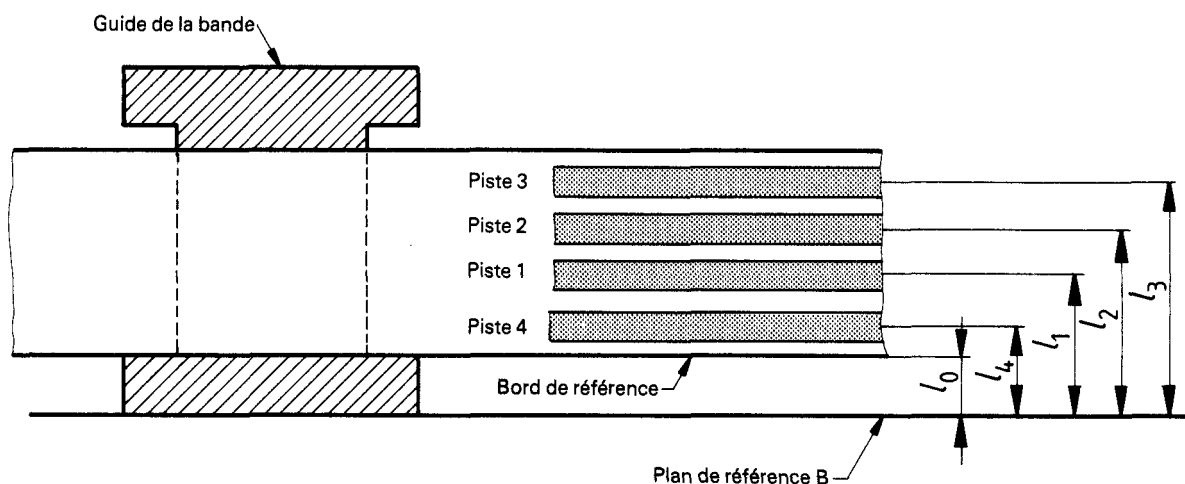
Figure 1 — Disposition des pistes
