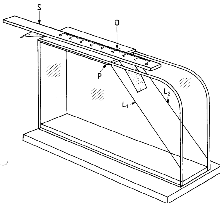
Figure D.1 — Flexomètre à angle fixe
