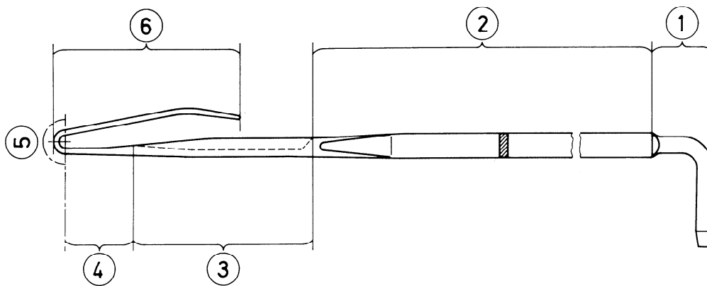
Figure 1 — Illustration showing the principal parts of a bearded needle Figure 1 — Illustration repérant les principales parties d'une aiguille à bec Чертеж 1 — Основные части крючковой иглы
