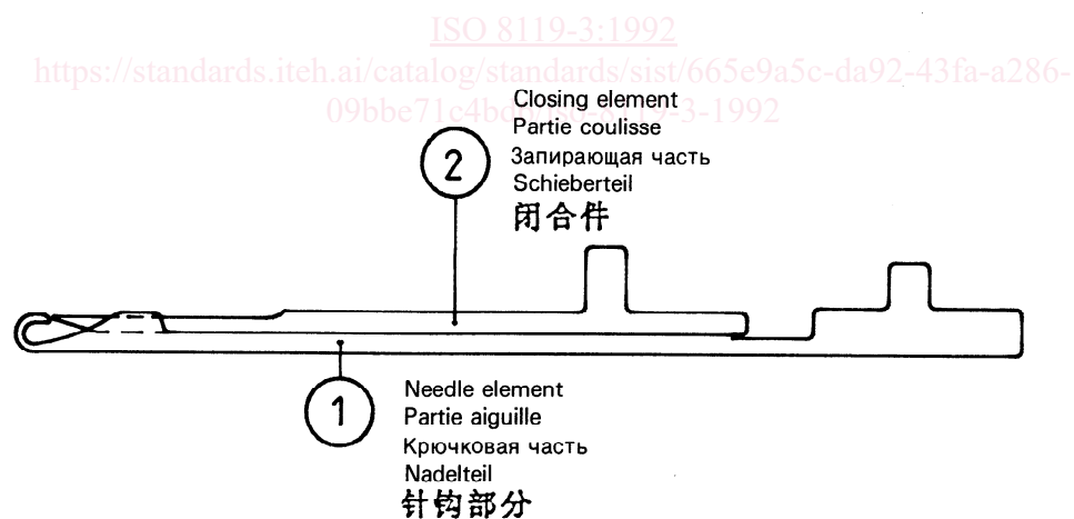
Figure 1 — Illustration showing the principal parts of a compound needle Figure 1 — Illustration repérant les principales parties d'une aiguille à coulisse Чертеж 1 — Иллюстрация, показывающая основные части движковой иглы
