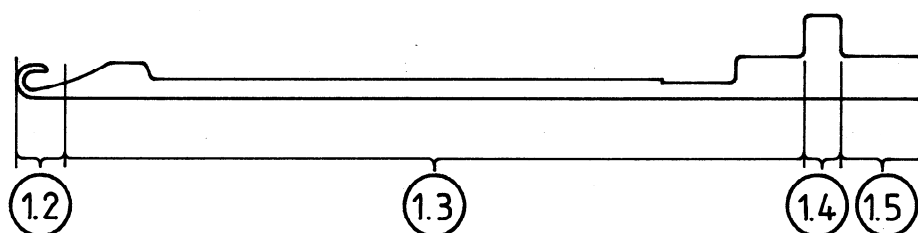
Figure 2 — Illustration showing the needle element in detail Figure 2 — Illustration repérant en détail la partie aiguille Чертеж 2 — Иллюстрация, показывающая крючковую часть
