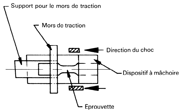
Figure 1 — Schéma montrant la relation entre le pendule et les mors pour la méthode A
