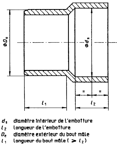
Figure 3 — Emplacement des points de mesure des emboîtures et des bouts mâles à collage au solvant
