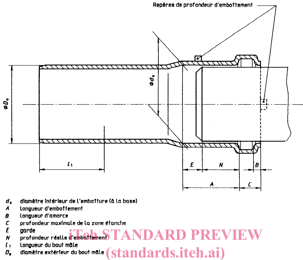
Figure 2 — Emplacement des points de mesure des emboîtures et des bouts mâles de type L
