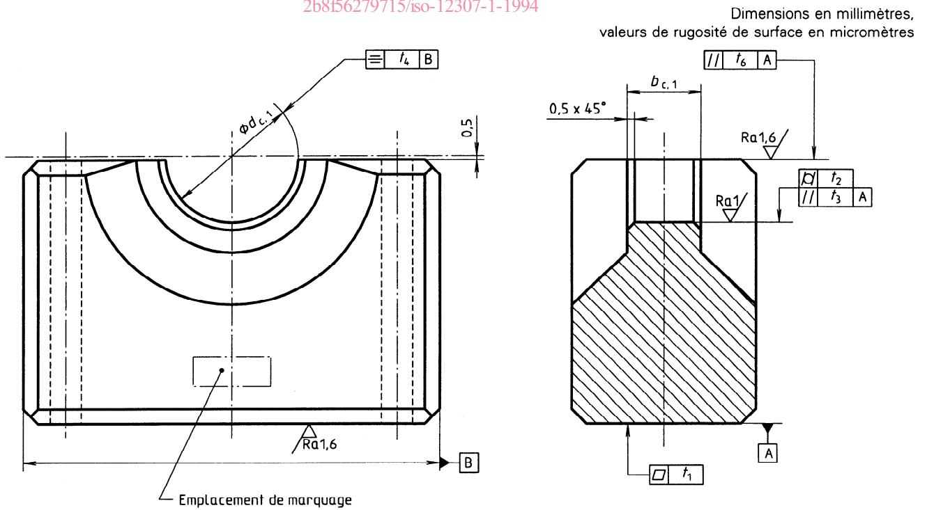
Figure 4 — Moitié inférieure du berceau de contrôle
