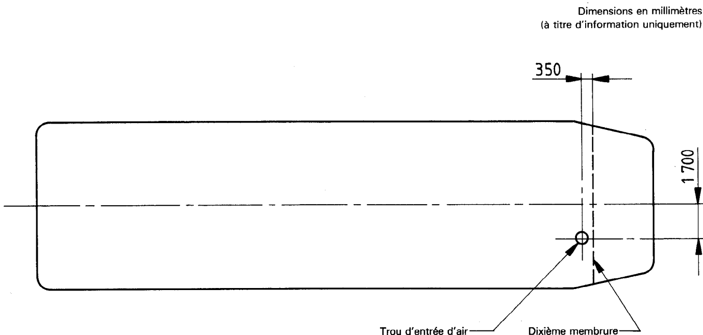
Figure 1 — Disposition du trou d'entrée d'air sur barge de la série 3 embarcable à bord d'un navire
