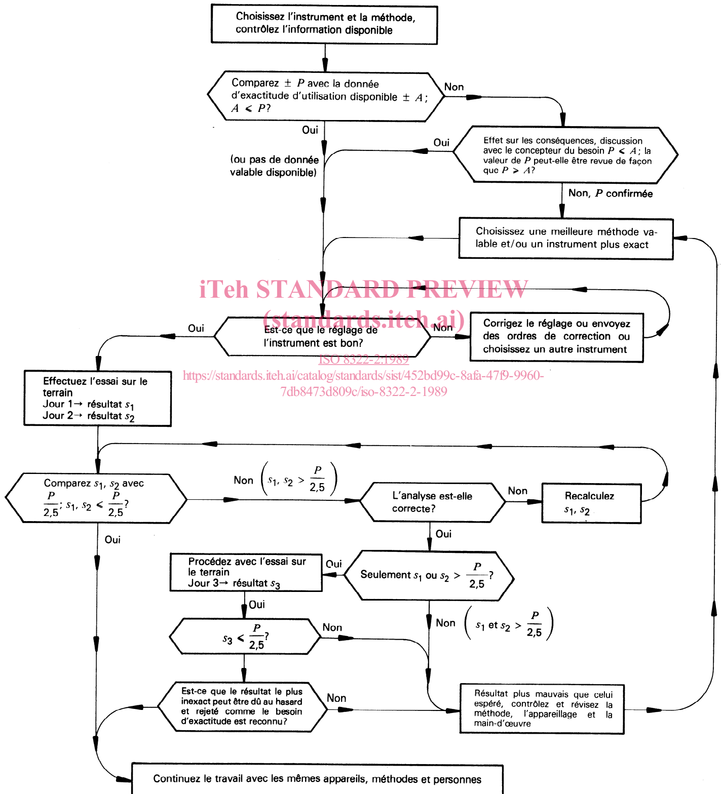
Figure 1 — Ordigramme pour les essais de l'exactitude d'utilisation
