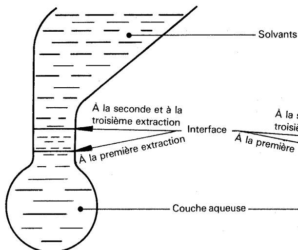
Figure 1 — Avant décantation (8.5.8, 8.5.12, 8.5.13)
