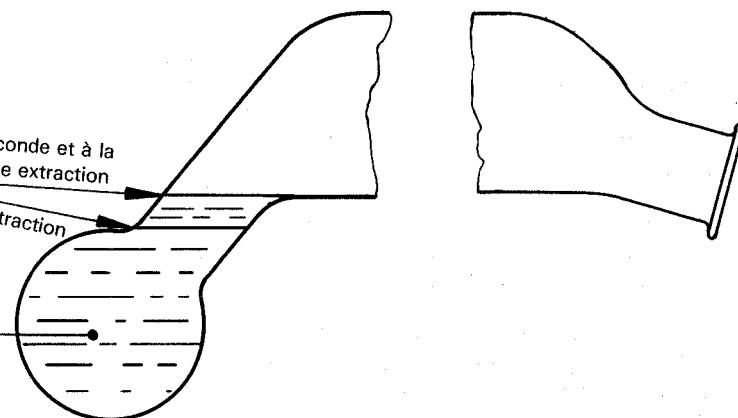
Figure 2 — Après décantation (8.5.9, 8.5.12, 8.5.13)
