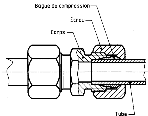
Figure 1 — Coupe transversale d'un raccord à compression type
