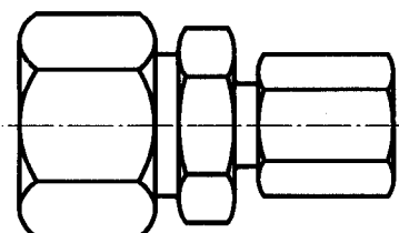
ISO 8434-1 - RES - S20 × S12
