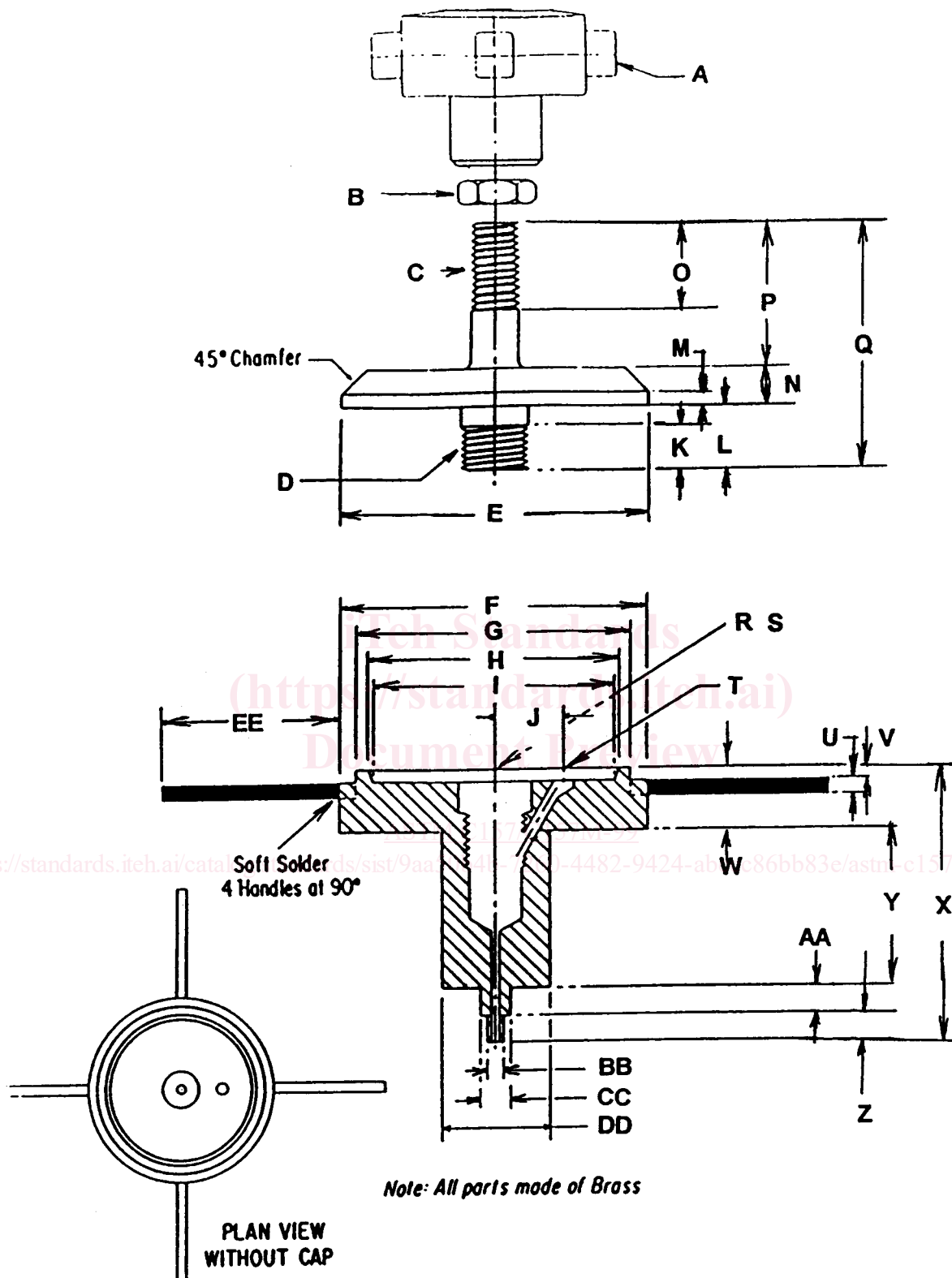
FIG. 1 Atmometer
