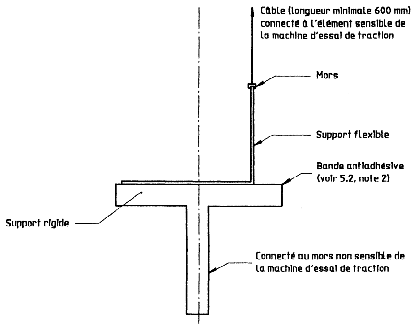
Figure 1 — Schéma de l'essai de pelage à 90° d'un assemblage collé flexible-sur-rigide
