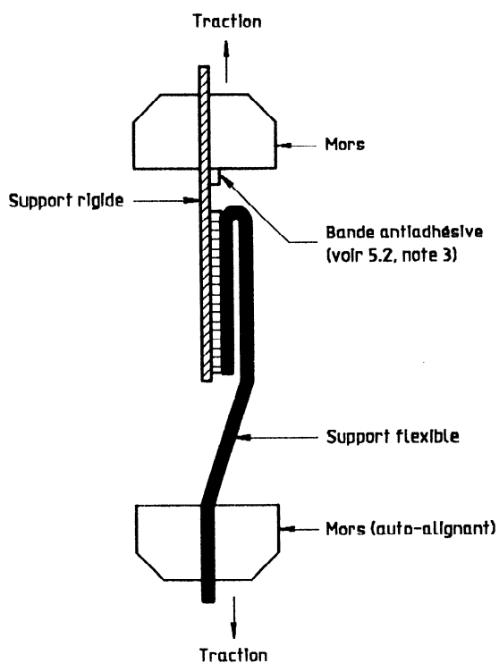
Figure 1 — Schéma de l'essai de pelage à 180° d'un assemblage collé flexible-sur-rigide (standards.iteh.ai)
