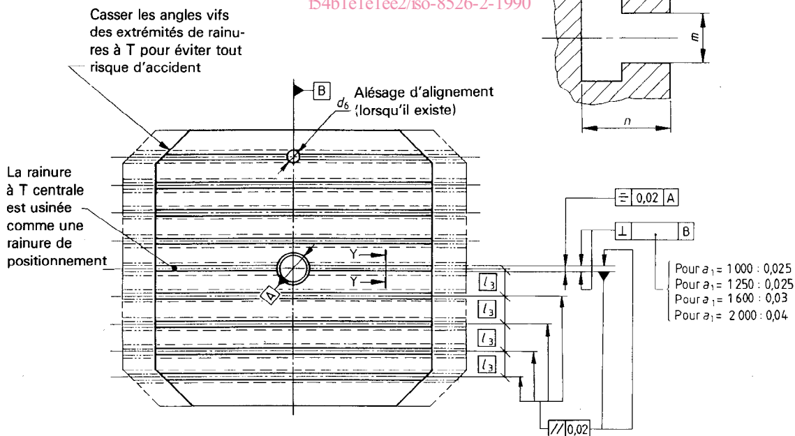
b) type 2, surface extérieure avec rainures à T
