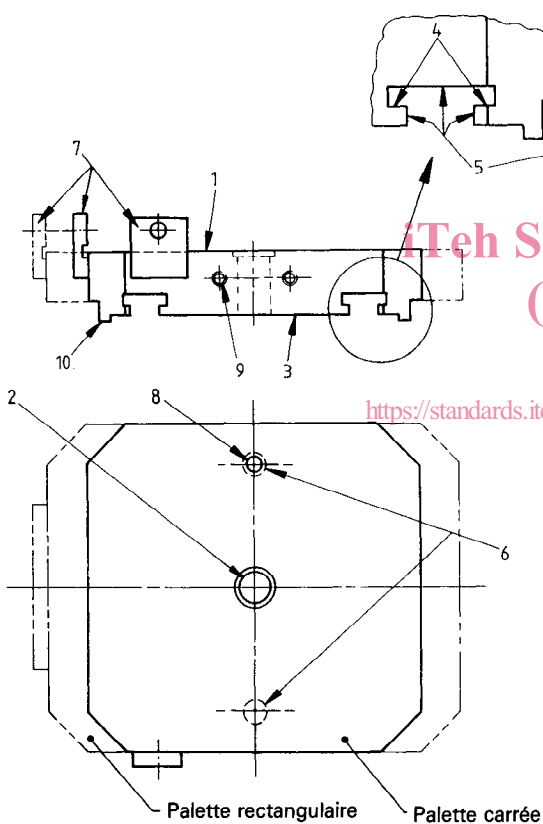
Figure 1 — Palette porte-pièce
