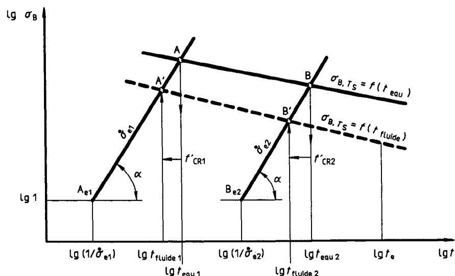
Figure A.1 — Représentation graphique de la droite de la contrainte de base d'un fluide
