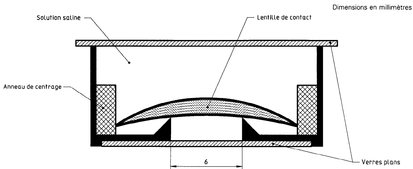
Figure 2 — Récipient utilisé pour mesurer le facteur de transmission des lentilles de contact dans une solution saline normalisée
