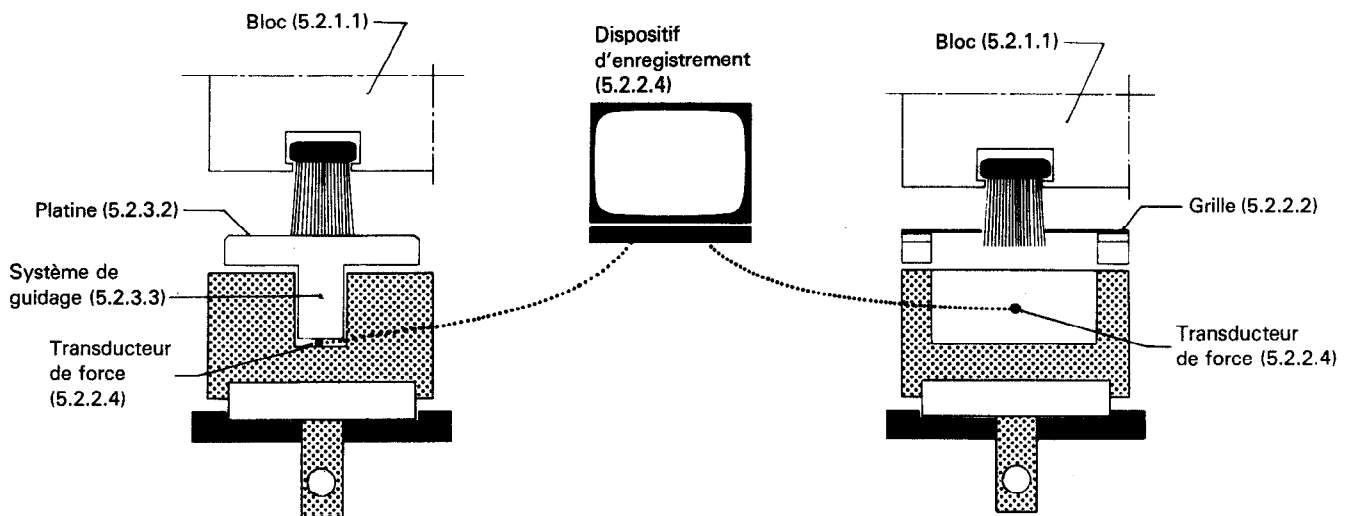
Figure — Schéma d'un appareillage convenable pour mesurer la dureté
