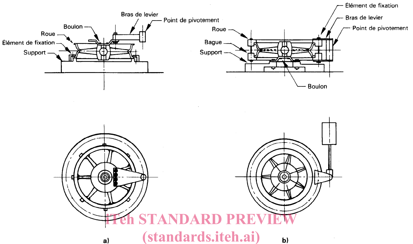
ISO 8645:1988 Figure 4 — Exemples d'équipement pour l'essai de torsion https://standards.iteh.ai/catalog/standards/sis/9509986-80-8010-1031-8095-11ab38e707d4/iso-8645-1988
