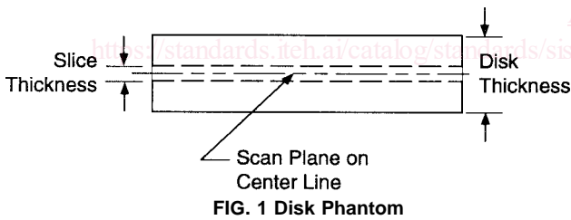
FIG. 1 Disk Phantom
