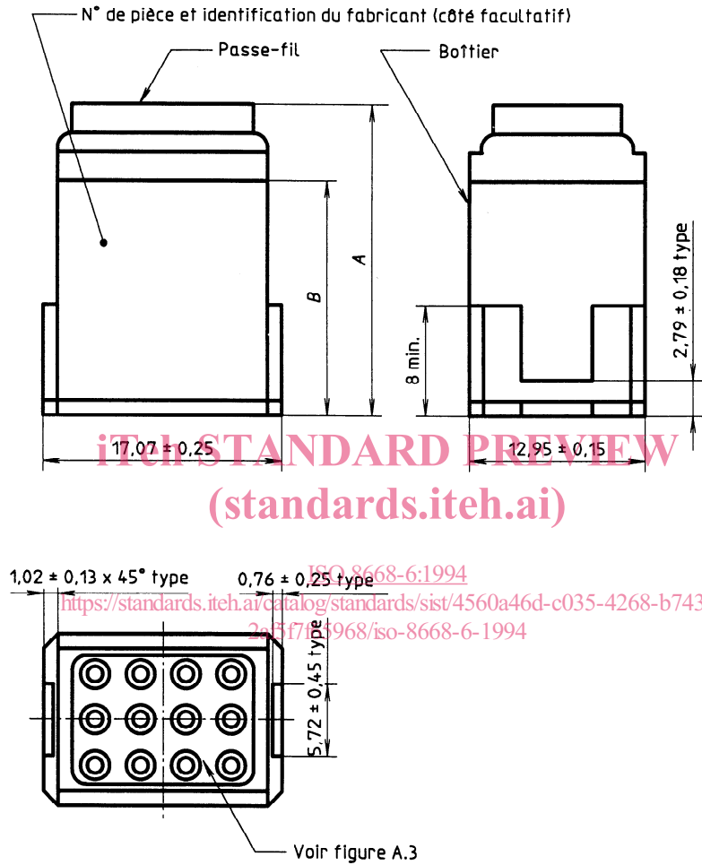
Figure A.1 — Modules des tailles 22, 20 et 16
