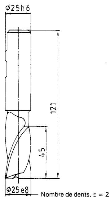
Figure 6 — Fraise à rainurer (voir ISO 1641-1)
