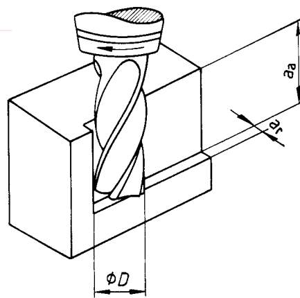
b) Fraisage en avalant
