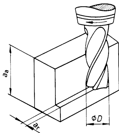
a) Fraisage en opposition
