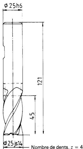
Figure 5 — Fraise 2 tailles (voir ISO 1641-1)
