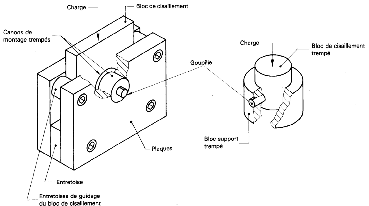
Figure — Montage-type pour l'essai de cisaillement des goupilles
