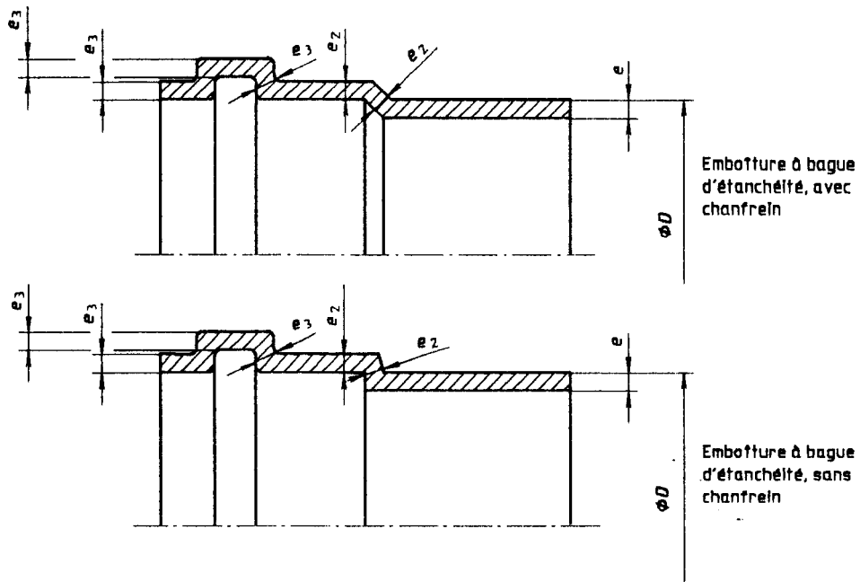
Figure 5 — Détails de l'emboîture (standards.iteh.ai)
