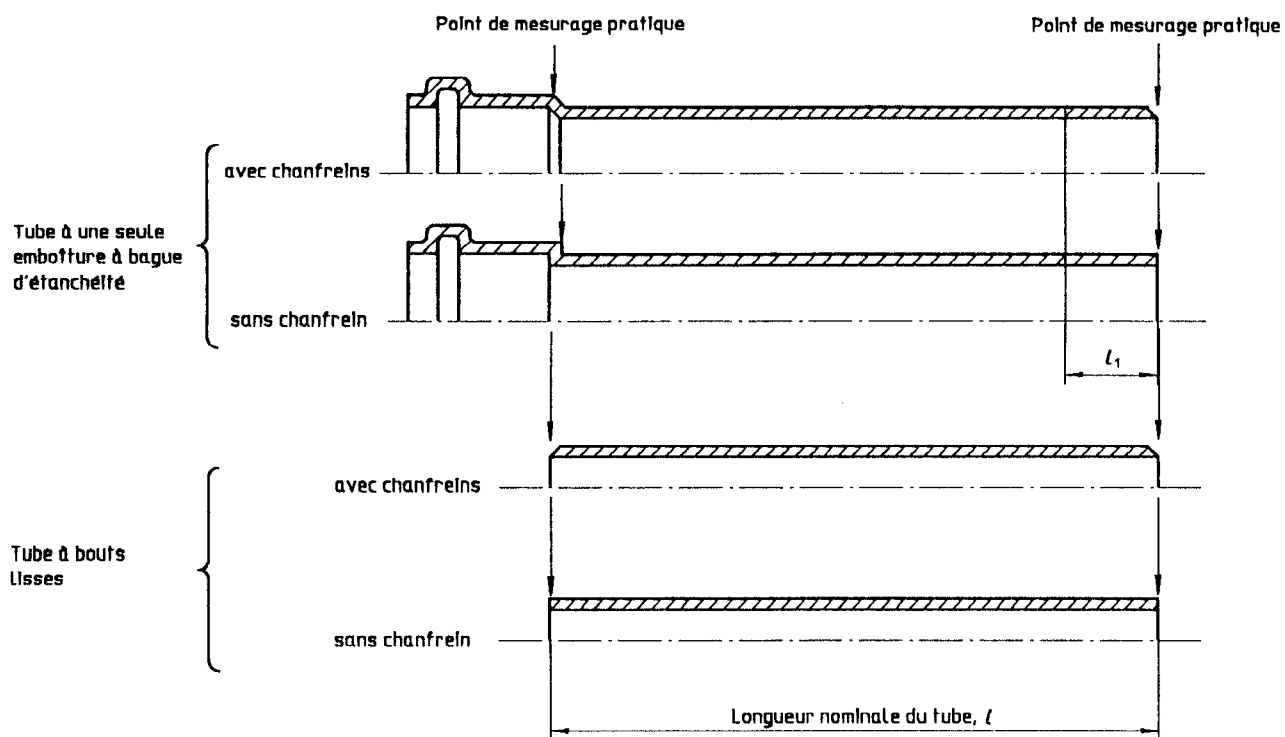
Figure 2 — Longueur nominale des tubes et définitions (standards.iteh.ai)
