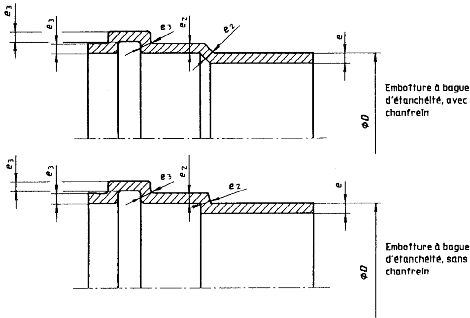
Figure 5 — Détails de l'emboîture iTeH STANDARD PREVIEW (standards.iteh.ai)
