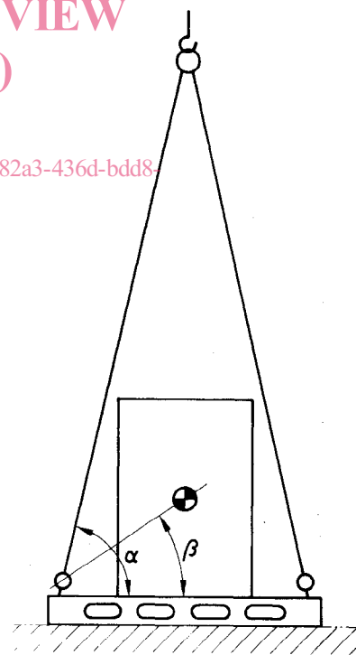
Figure 4 – Exemple d'un centre de gravité d'une charge situé plus haut que les points d'accrochage
