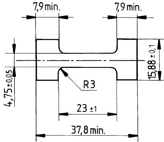
Figure 1 — Éprouvette pour l'essai de traction
