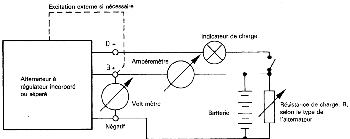
Figure 1 — Schéma pour l'essai de l'alternateur
