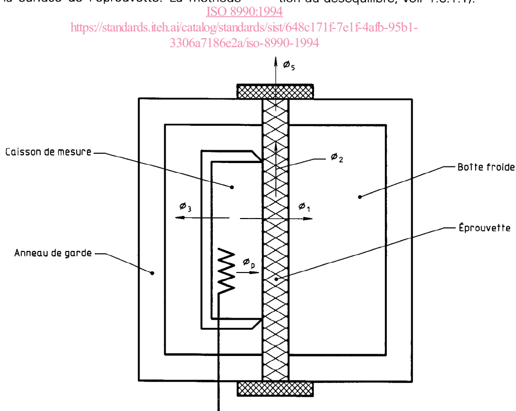
Figure 1 — Boîte chaude gardée
