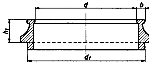
Dimensions en millimètres
