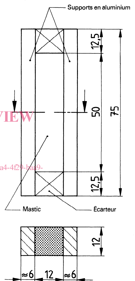
Figure 2 – Éprouvette avec supports en aluminium
