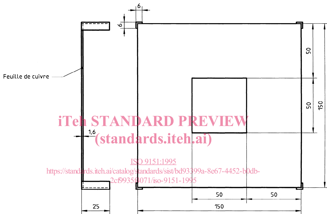
Figure 3 — Porte-éprouvette
