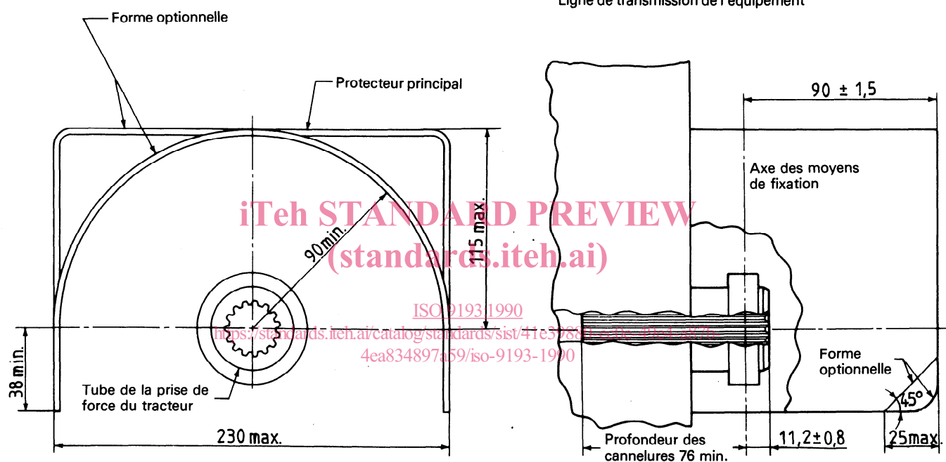
Figure 1 — Dimensions des moyens de fixation de la prise de force et du protecteur principal
