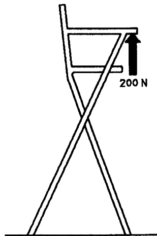
Figure 3 — Essai de pilage des chaises hautes
