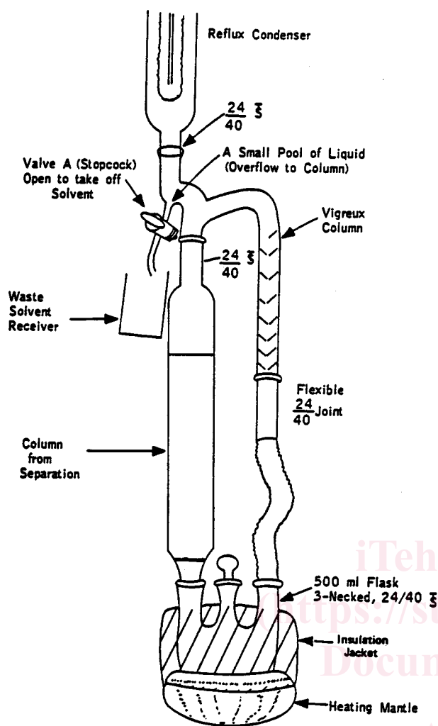
FIG. 2 Extraction Apparatus
