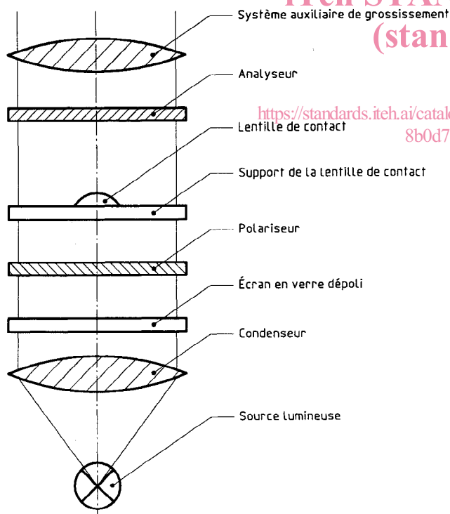
Figure A.1 — Dispositif de mesure
