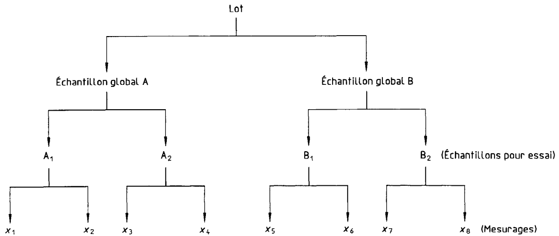
Figure 3 — Schéma de procédure de préparation/essai de type 1
