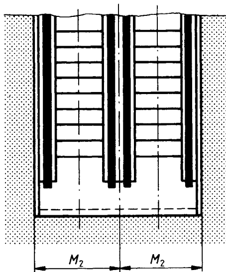
Figure 2 — Disposition en parallèle ou croisée
