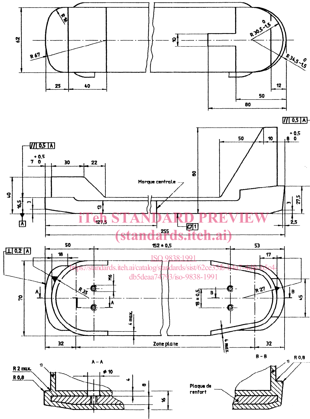
Figure 2 — Semelle d'essai type C
