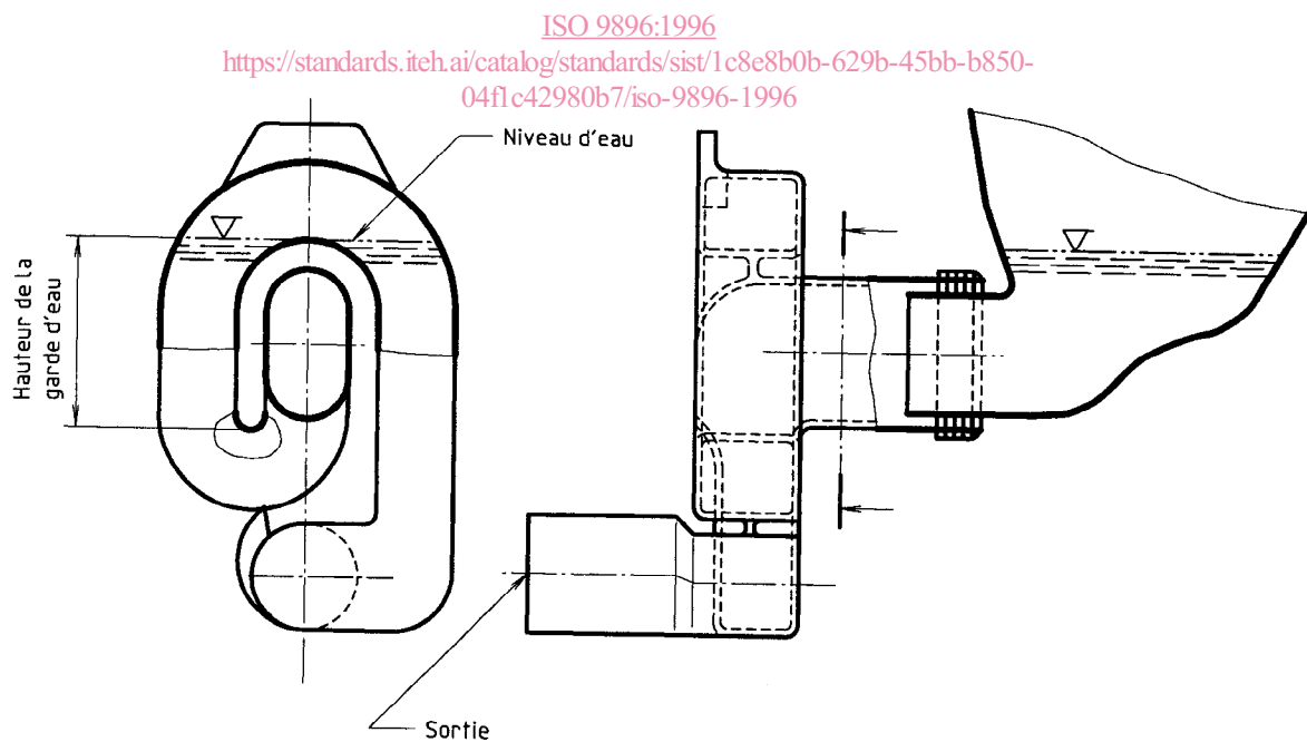
Figure 4 — Siphon d'urinoir
