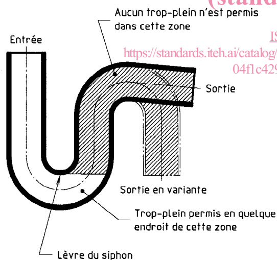
Figure 6 — Positions des orifices d'entrée et de sortie
