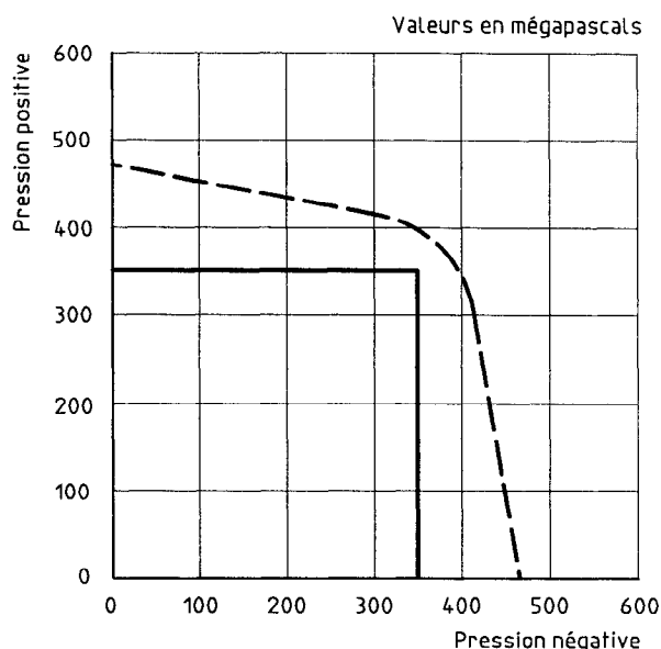
Figure 7 — Diagramme de la conservation de la garde d'eau
