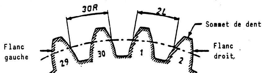
Figure 1 : Notation et numérotation d'une roue à denture extérieure 30R = pas n°30, flanc droit 2L = pas n°2, flanc gauche
