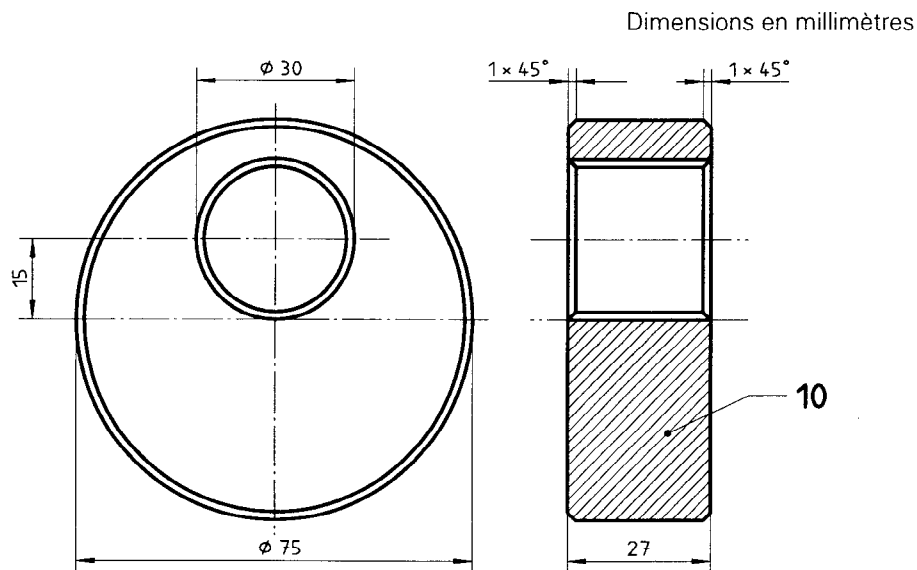
Figure 4 — Disques déséquilibres
