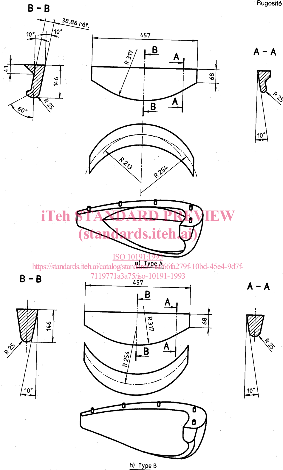
Figure 1 — Schémas des sabots de décoincement du talon
