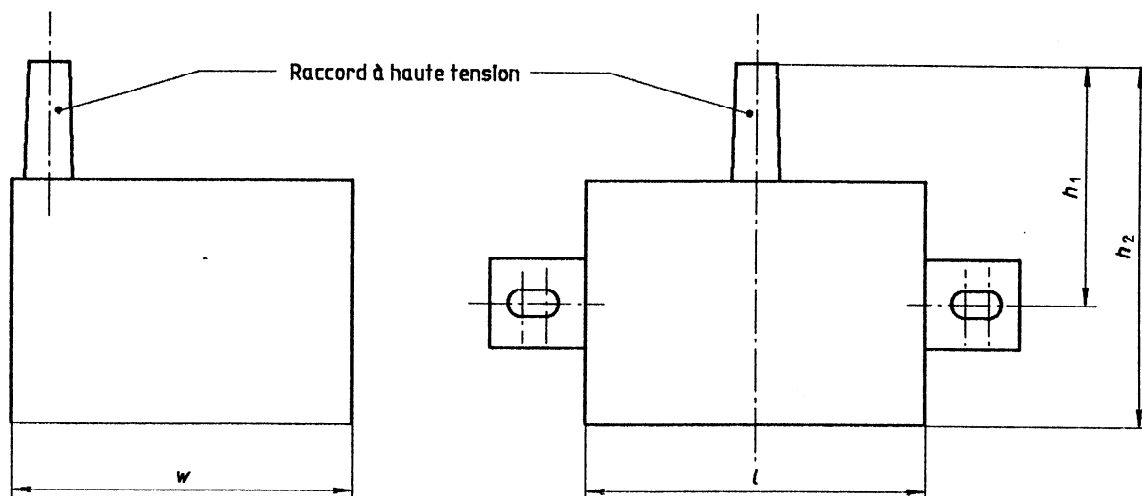
Figure 4 — Dimensions hors tout des bobines d'allumage à pattes de fixation (standards.iteh.ai)
