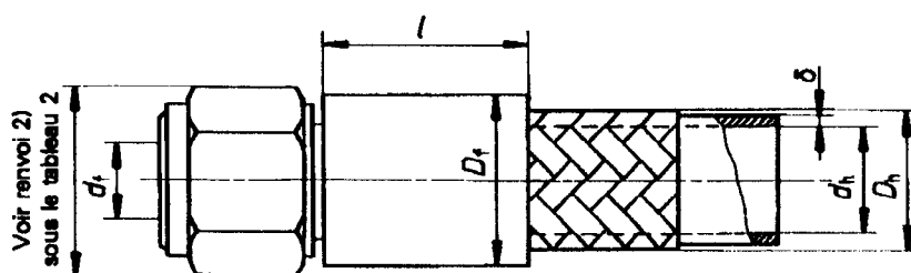
Figure 1 — Dimensions du tuyau flexible et des raccords
