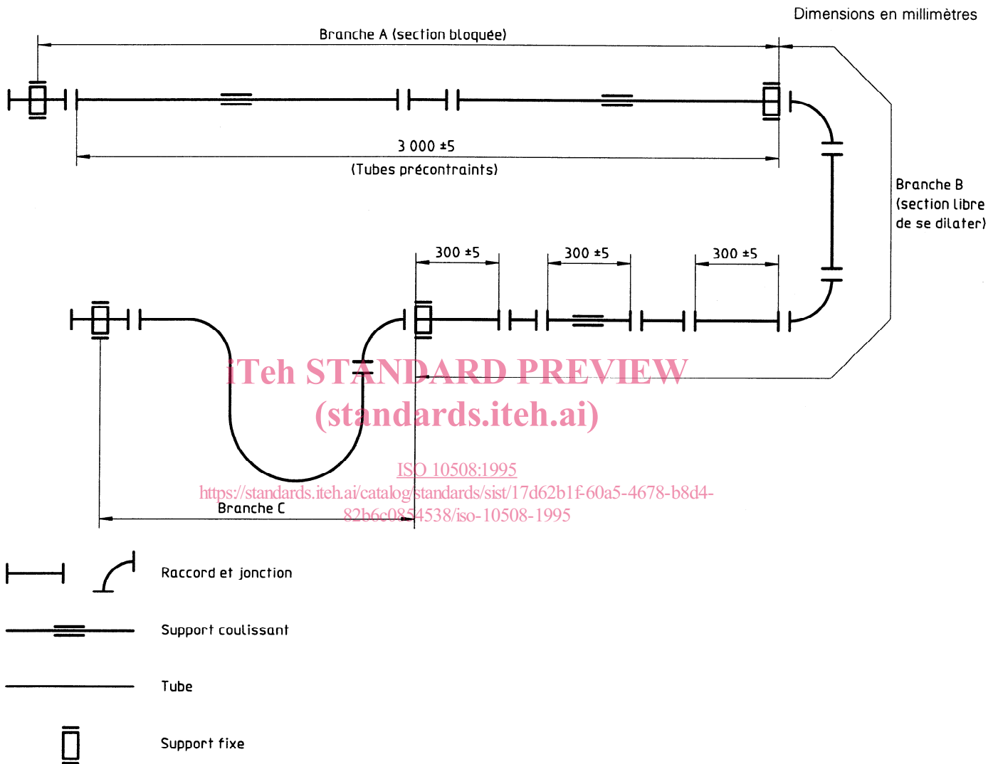
Figure A.1 — Assemblage d'essai pour les systèmes comportant des tubes souples
